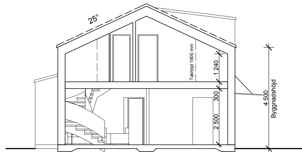
SEKTION A-A
