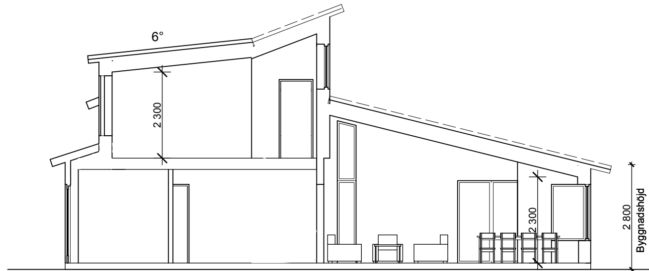
SEKTION A-A
