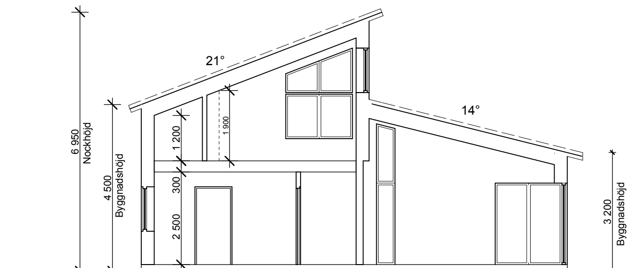
SEKTION B-B
